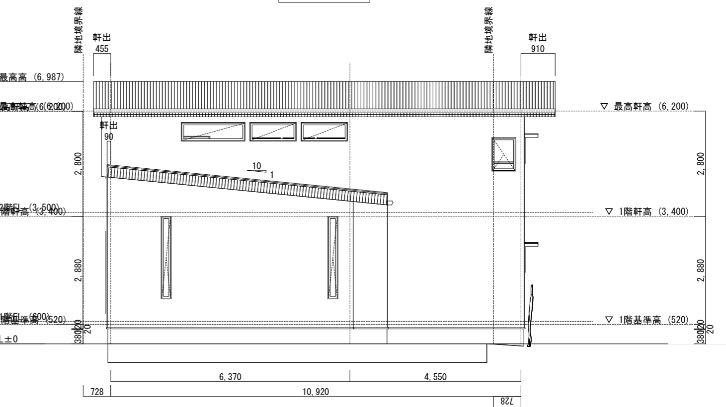
東立面図
