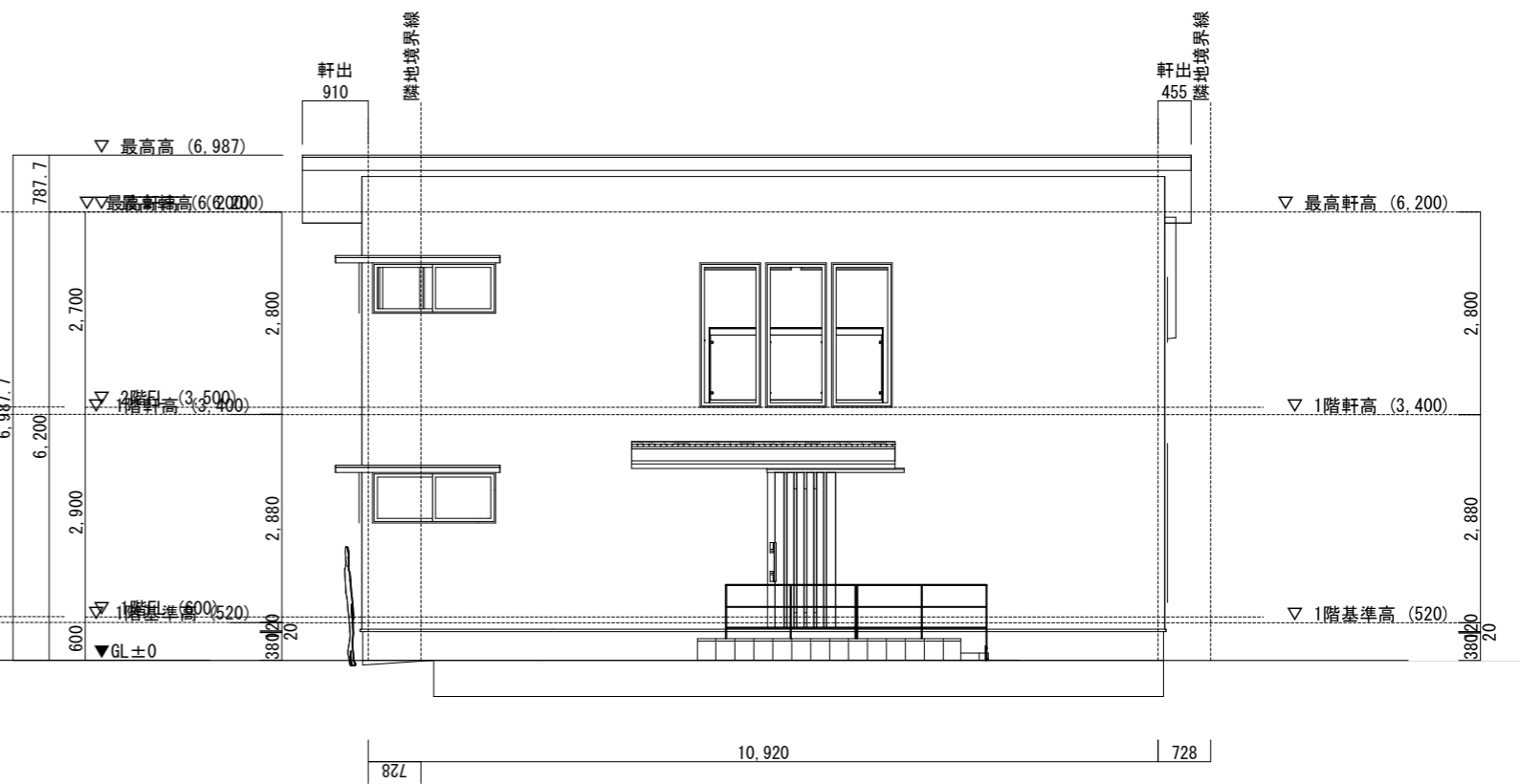
東立面図
