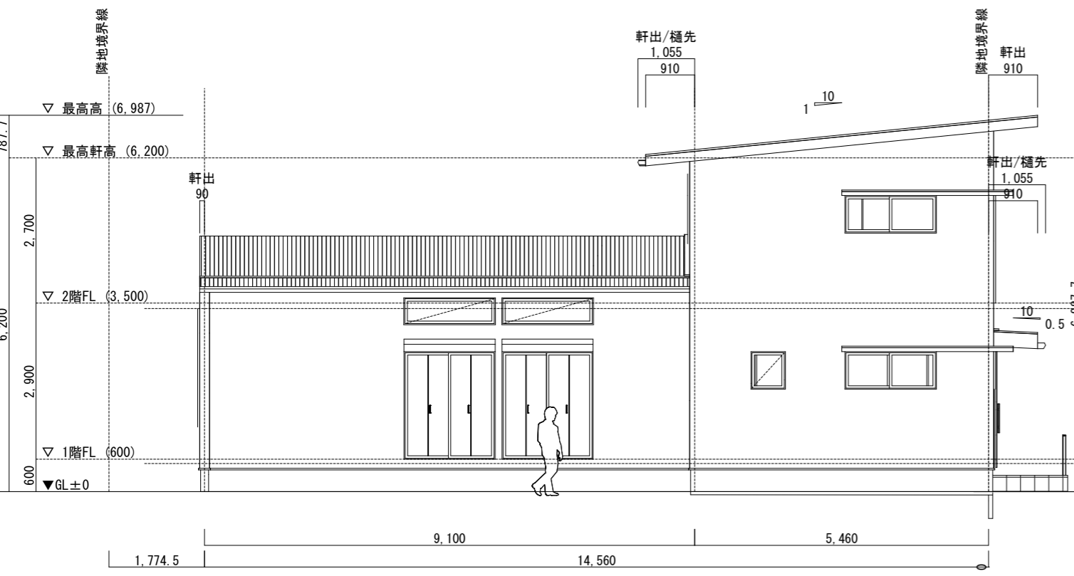
南立面図
