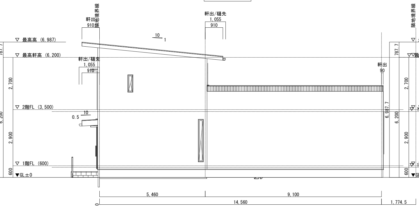
南立面図
